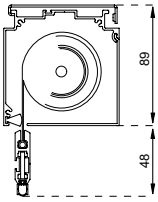
Fondale 11x41 (rullo guidata)
