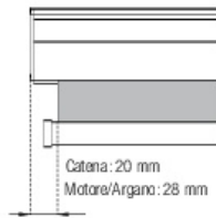
Tolleranza laterale del tessuto: catena 20mm
