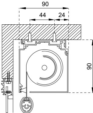
Montaggio a soffitto con supporto
