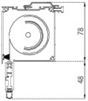
Fondale 11x41 (rullo guidata)
