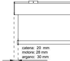
Tolleranza laterale del tessuto: motore 28mm - argano 30mm
