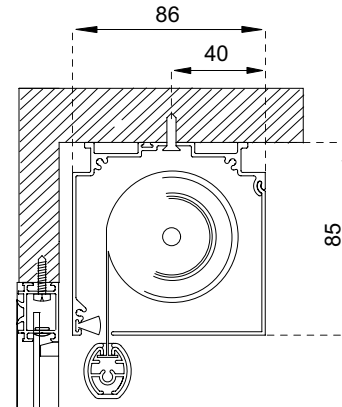
Montaggio a soffitto/parete diretto
