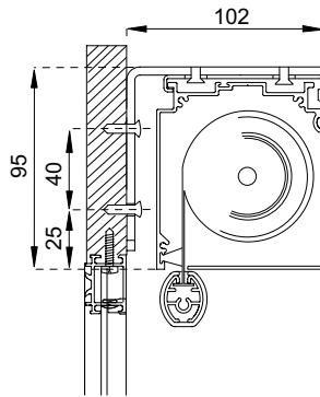
Montaggio a parete con staffa
