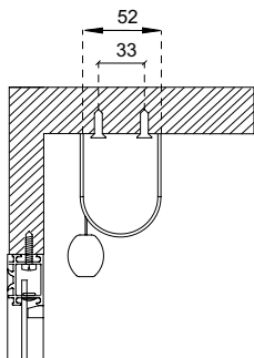
Montaggio a soffitto
