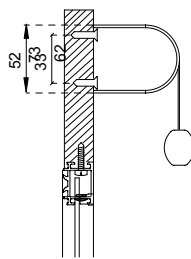
Montaggio a muro
